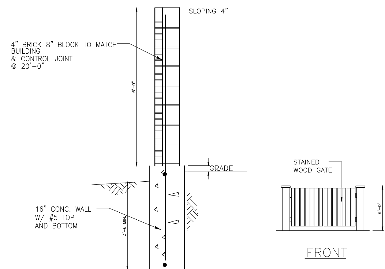
NEW DUMPSTER WALL DETAIL N.T.S.
